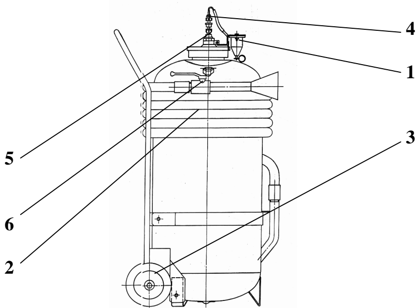
Внешний вид огнетушителя
